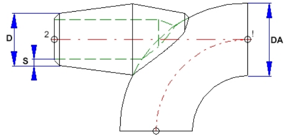
Beispiel Elbolet
