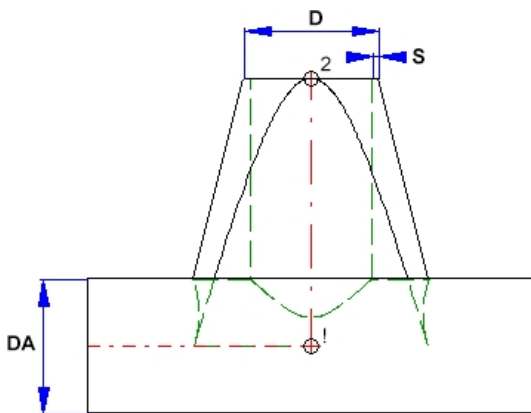
Beispiel Sattelstutzen
