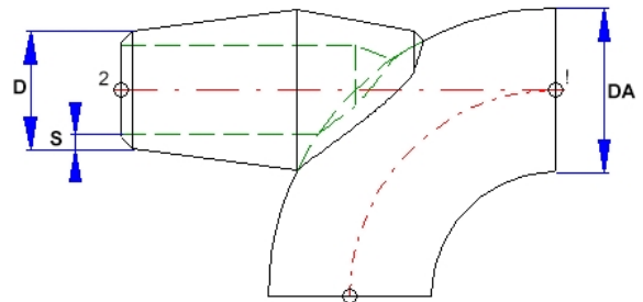
Beispiel Elbolet
