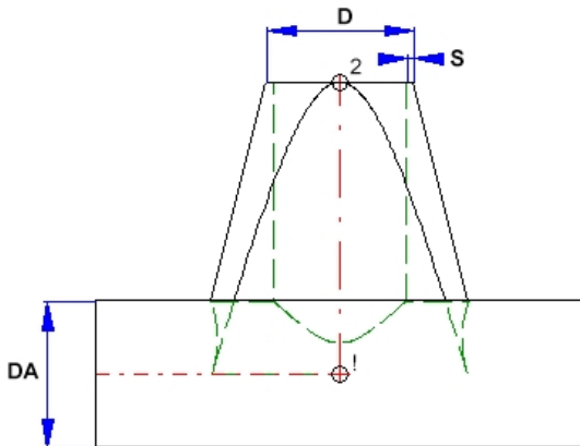
Beispiel Sattelstutzen
